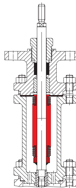
Сифонное уплотнение с защитным сальником
