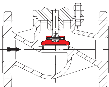
Запорный затвор
